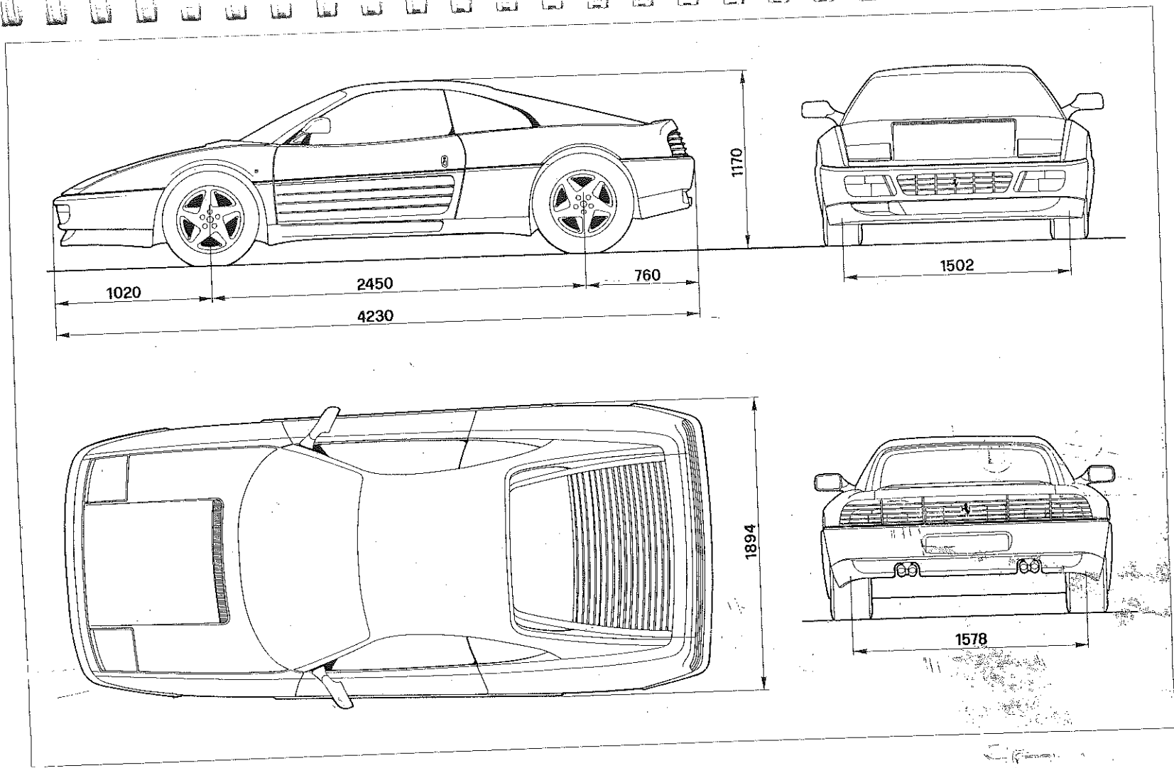
Abb. 1 - Fahrzeugmaße
