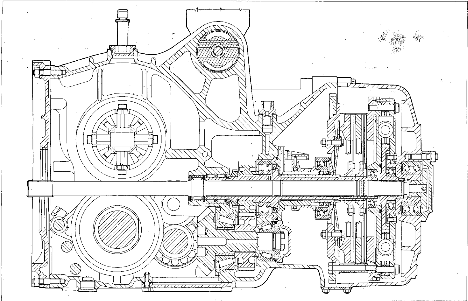
Fig. 5 - Complesso frizione - cambio - differenziale (Sezione longitudinale)
