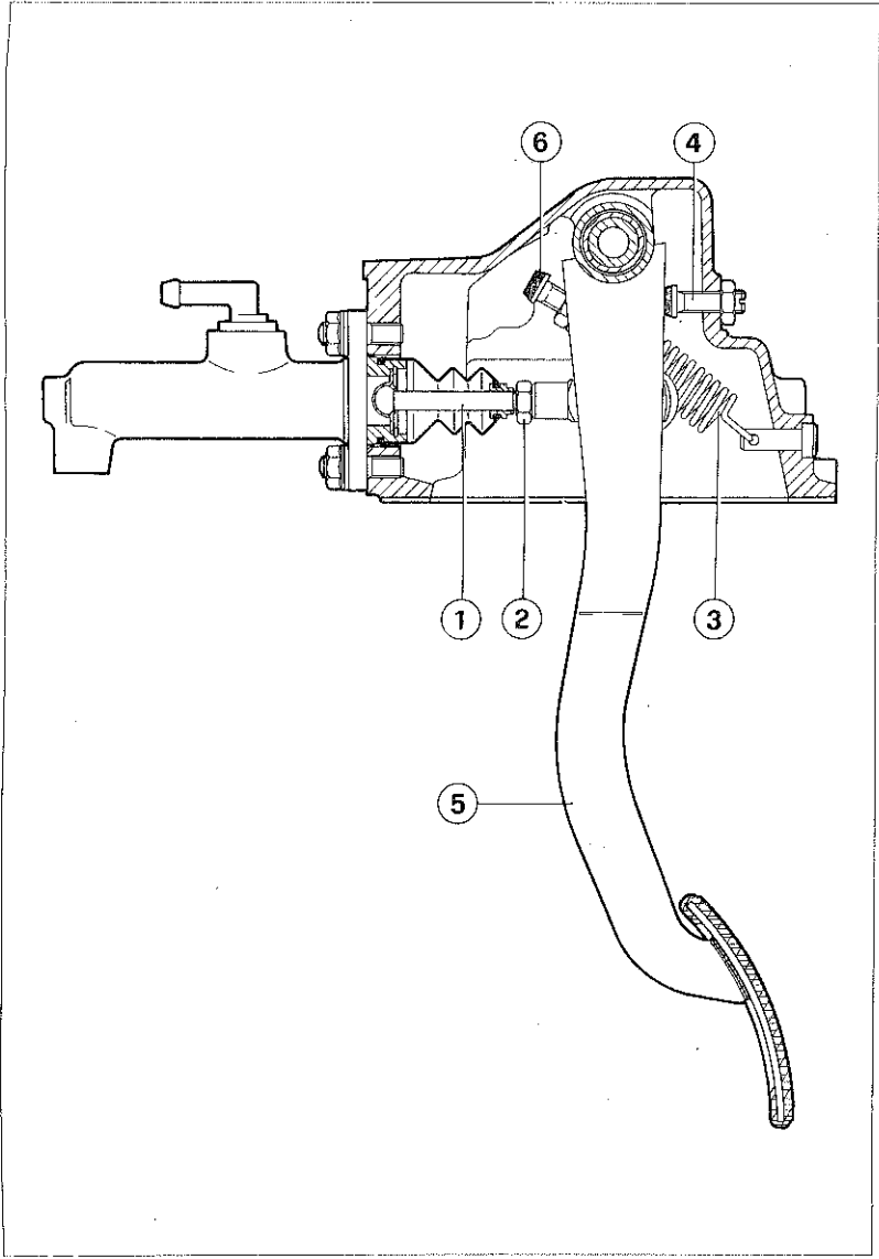
1) Pedaliera comando frizione 1 - Puntalino; 2 - Dado; 3 - Molla richiamo pedale; 4 - Puntalino registrazione allineamento pedale; 5 - Pedale frizione; 6 - Puntalino registrazione corsa pedale; 2) Sezione longitudinale frizione
