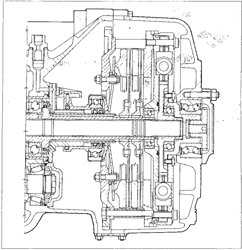
1) Pedaliera comando frizione 1 - Puntalino; 2 - Dado; 3 - Molla richiamo pedale; 4 - Puntalino registrazione allineamento pedale; 5 - Pedale frizione; 6 - Puntalino registrazione corsa pedale; 2) Sezione longitudinale frizione
