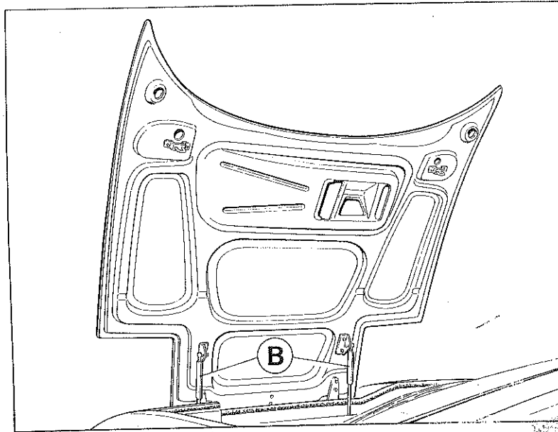
Fig. 22 - 23 - 24 - Capot avant A - Levier d'ouverture capot; B - Amortisseurs soutien capot; C - Anneau d'ouverture de secours.
